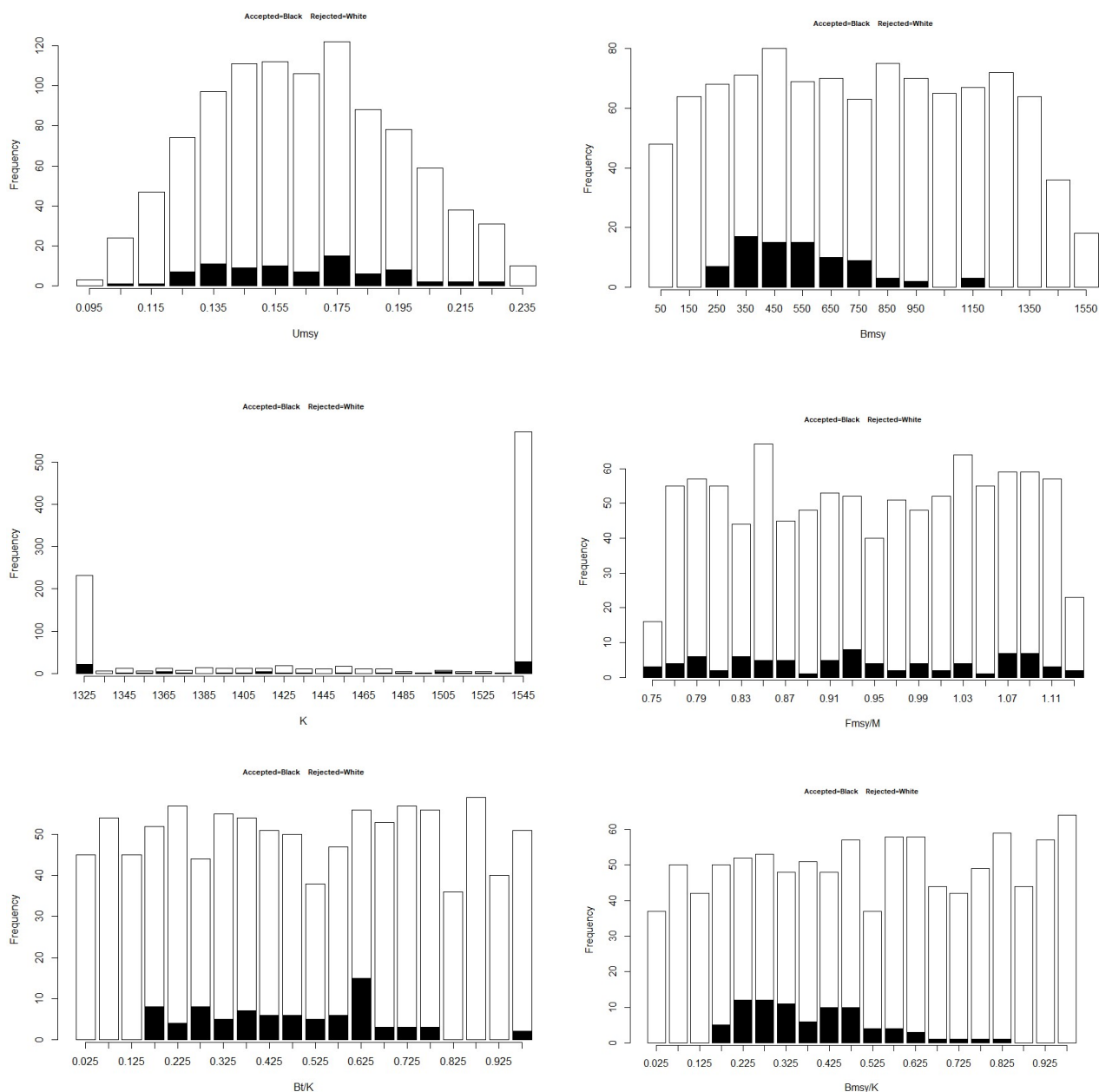
Рис. 3.19. Принятые и отвергнутые параметры для построения траекторий биомасс
