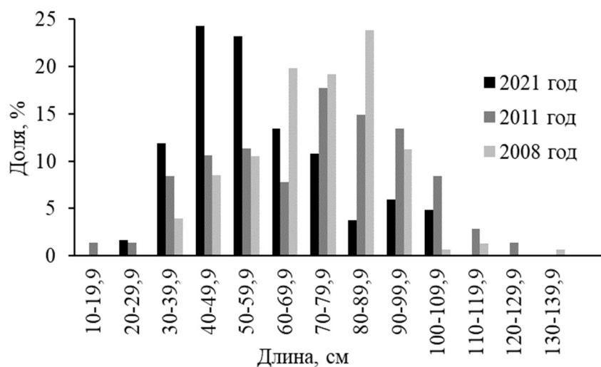
Рис. 6.6. Размерный состав уловов амурского осетра в реке Амур
