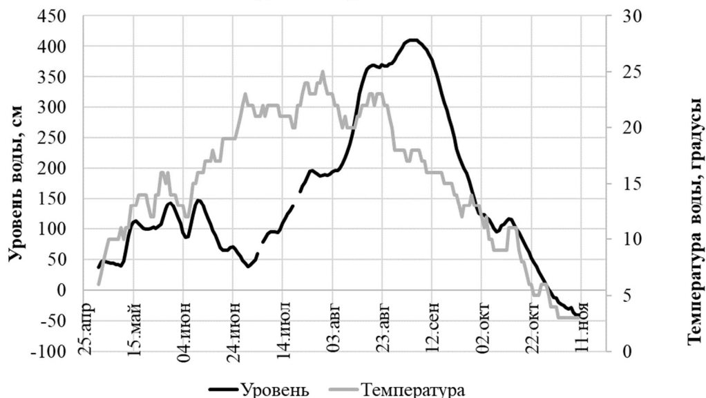
Рис. 2.16. Сезонная динамика уровня и температуры воды в бассейне Амура по створу г. Хабаровск в 2023 г.
