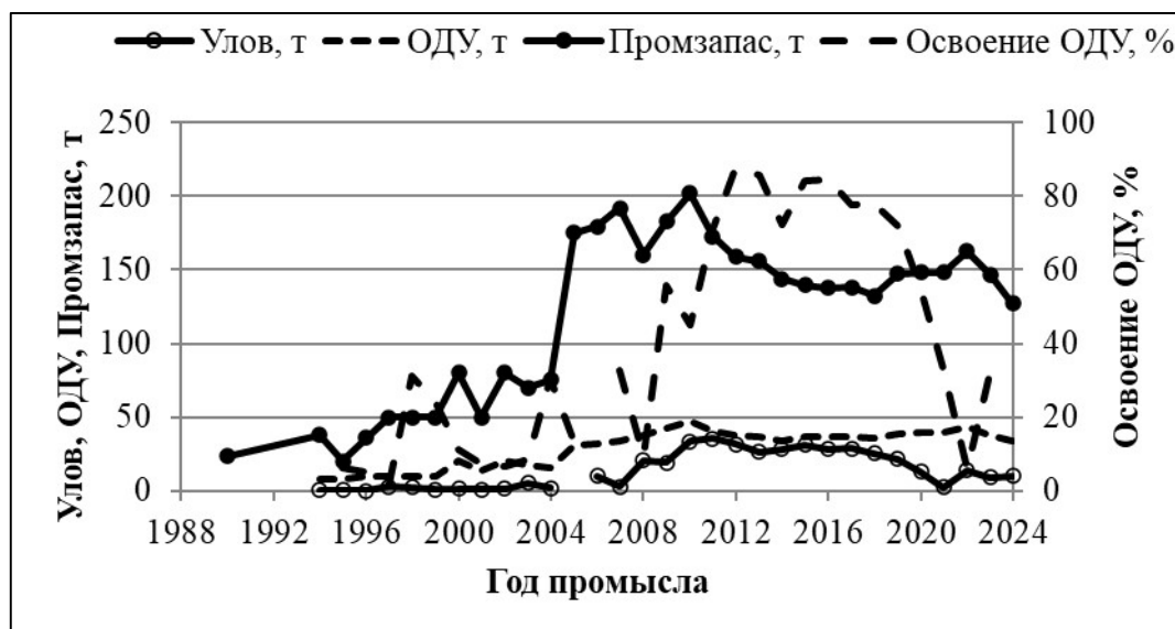
Рис. 3.6. Динамика уловов, ОДУ, промыслового запаса и освоение ОДУ, % амурского белого леща в бассейне р. Амур на территории Хабаровского края и ЕАО
