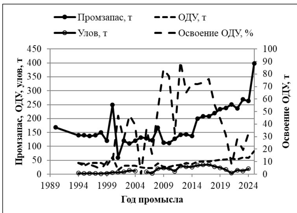
Рис 3.15. Динамика уловов, ОДУ, промыслового запаса (т) и освоение ОДУ (%) сома в пределах Хабаровского края и ЕАО
