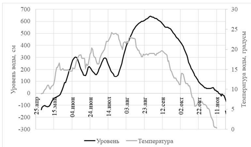
Рис. 2.12. Сезонная динамика уровня и температуры воды в бассейне Амура по створу г. Хабаровск в 2019 г.
