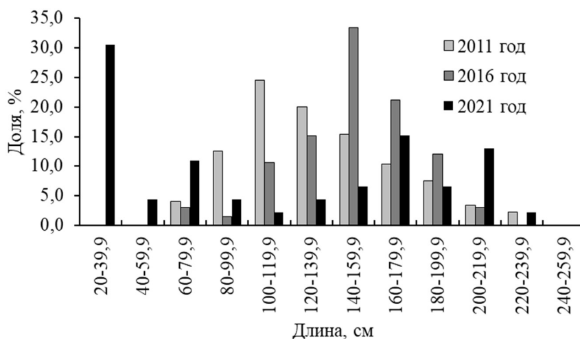
Рис. 6.13. Распределение калуги по длине, лиман Амура
