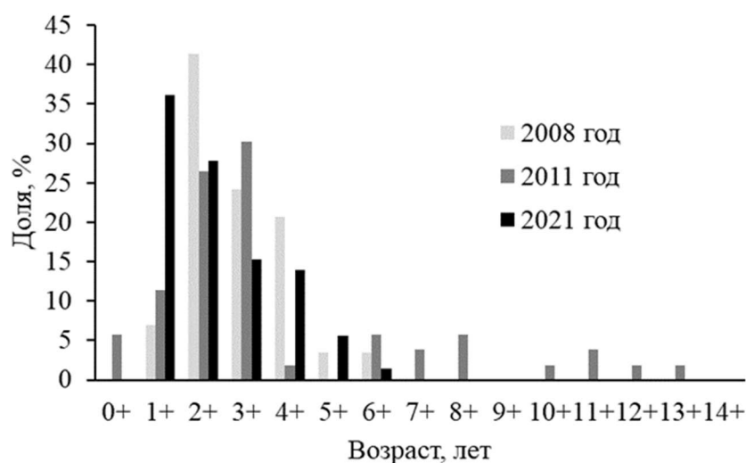
Рис. 6.15. Возрастной состав уловов калуги в реке Амур
