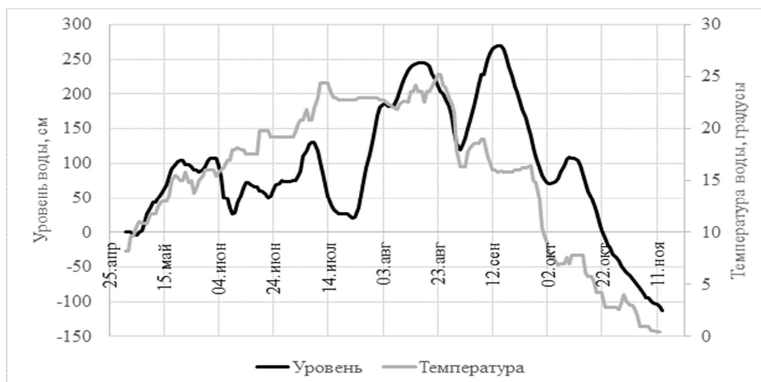
Рис. 2.10. Сезонная динамика уровня и температуры воды в бассейне Амура по створу г. Хабаровск в 2017 г.
