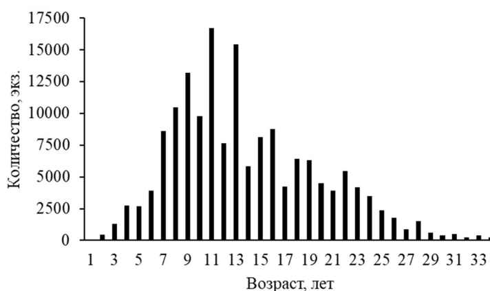
Рис. 6.5. Возрастной состав уловов амурского осетра в Амурском лимане в 2021 г.
