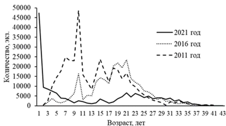
Рис. 6.14. Возрастной состав уловов калуги в Амурском лимане
