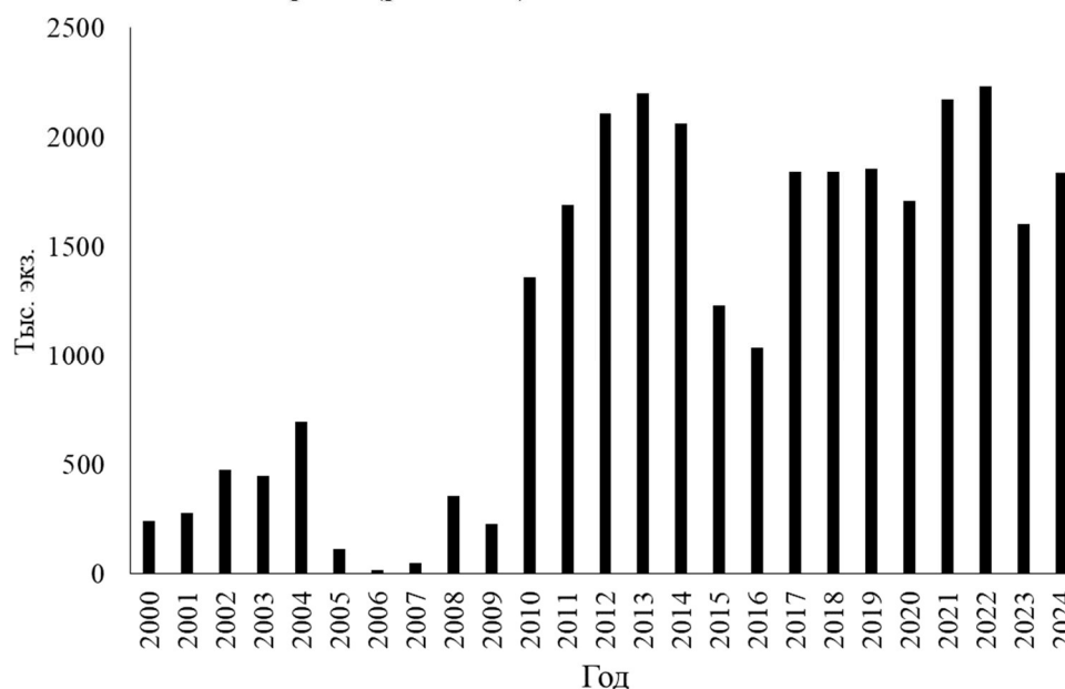
Рис. 6.8. Объемы выпуска молоди амурского осетра в 2000-2024 гг.
