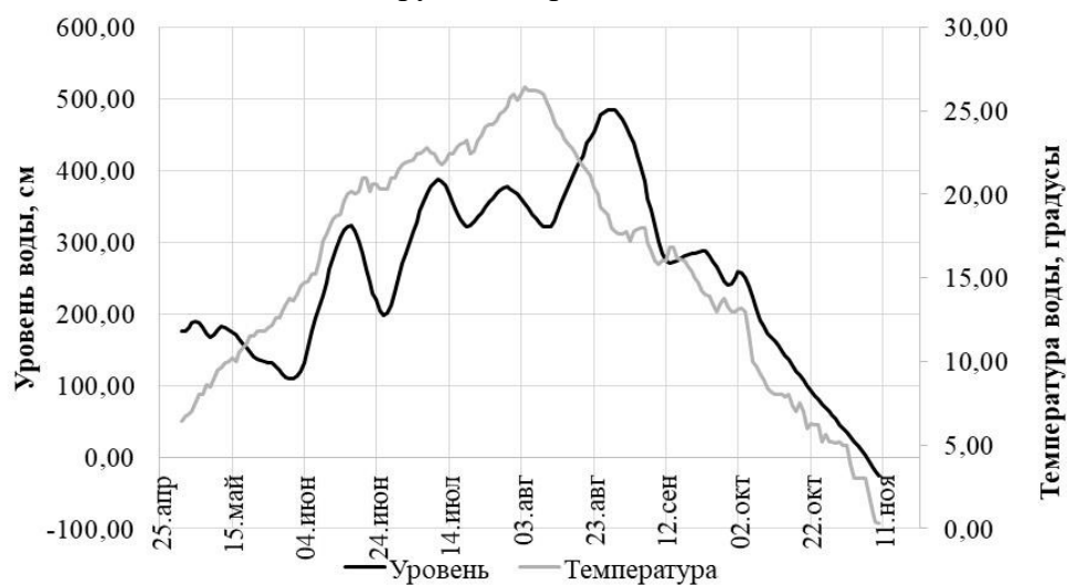
Рис. 2.14. Сезонная динамика уровня и температуры воды в бассейне Амура по створу г. Хабаровск в 2021 г.
