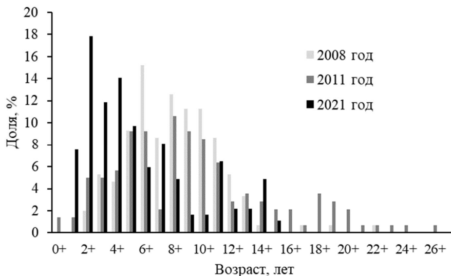
Рис. 6.7. Возрастной состав уловов амурского осетра в реке Амур
