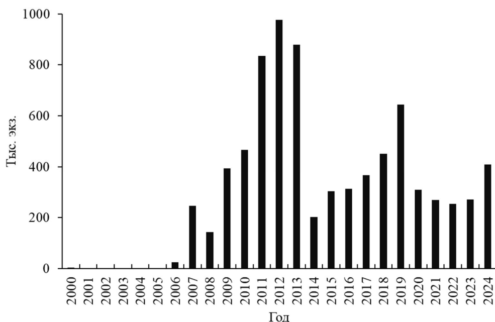
Рис. 6.16. Объемы выпуска молоди калуги в последние 20 лет.
