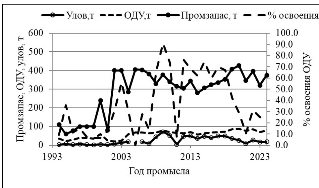
Рис. 3.3. Динамика промыслового запаса (т), ОДУ (т), вылова (т) и % освоения ОДУ верхогляда в бассейне р. Амур на территории ЕАО и Хабаровского края
