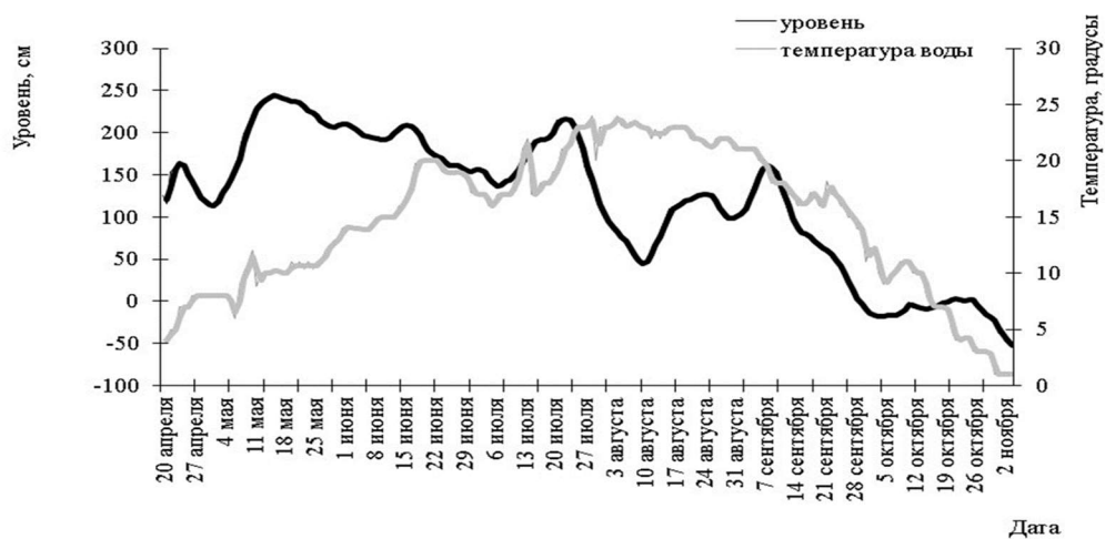
Рис. 2.8. Сезонная динамика уровня и температуры воды в бассейне Амура по створу г. Хабаровск в 2015 г.
