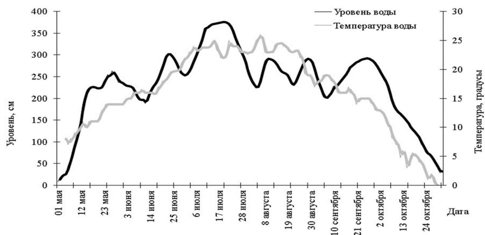
Рис. 2.9. Сезонная динамика уровня и температуры воды в бассейне Амура по створу г. Хабаровск в 2016 г.
