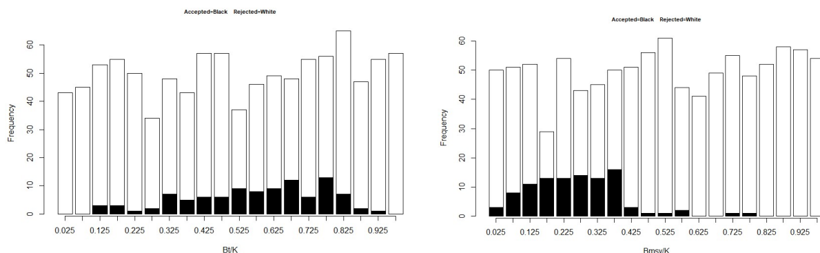
Рис. 3.4. Принятые и отвергнутые параметры для построения траекторий биомасс.
