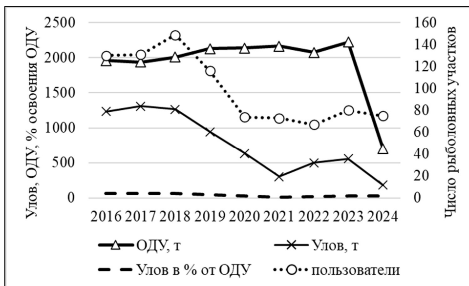
Рис. 2.6. Уловы пресноводных рыб и число РЛУ на промысле пресноводных рыб бассейна р. Амур (Хабаровский край и ЕАО) в период с 2016 по 2024 гг.
