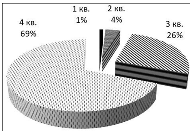
Рис. 3.17. Динамика годового вылова амурской щуки, %
