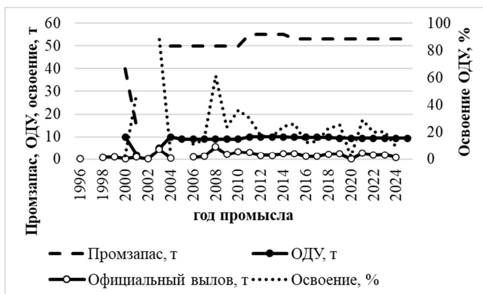
Рис. 3.22. Динамика промыслового запаса, ОДУ, уловов (т) и освоения ОДУ (%) тайменей р. Амур
