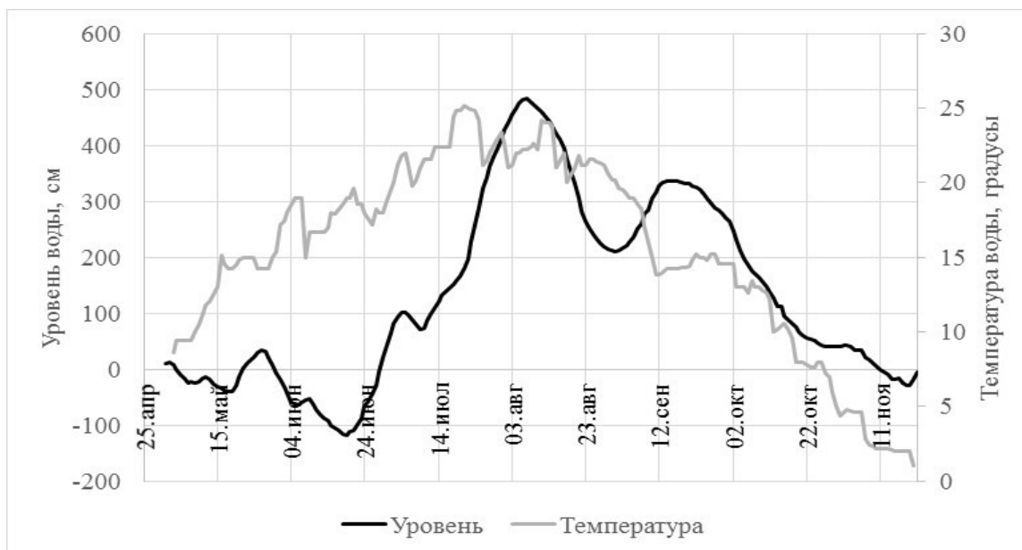
Рис. 2.11. Сезонная динамика уровня и температуры воды в бассейне Амура по створу г. Хабаровск в 2018 г.
