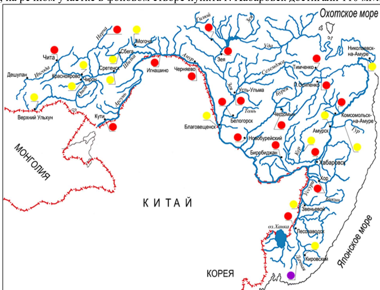
Рис. 2.18. Комплексная оценка качества поверхностных вод бассейна р. Амур в 2023 г.
