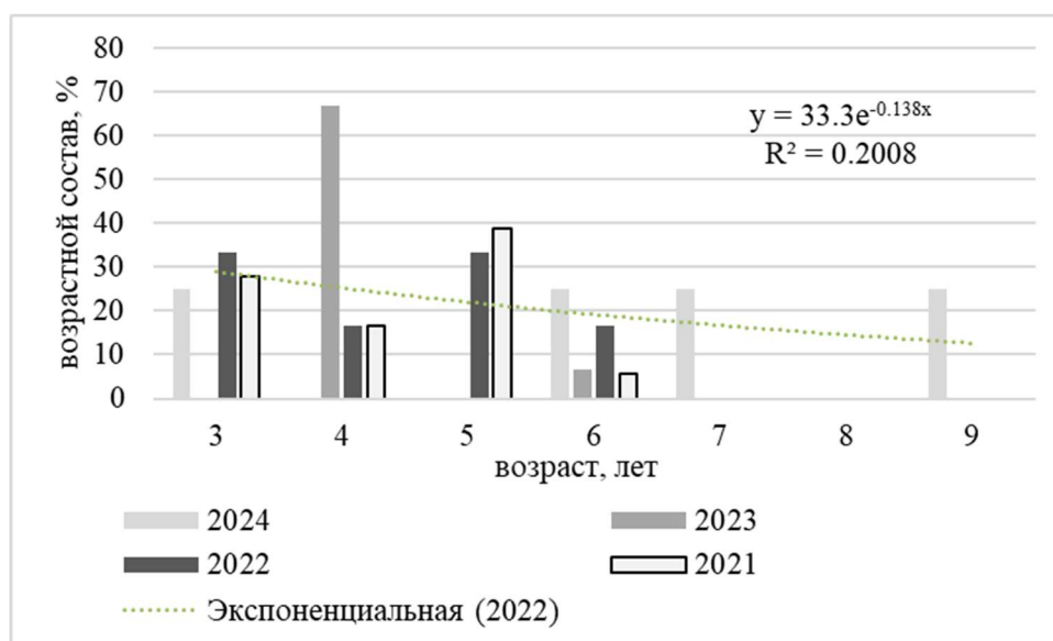
Рис. 3.23. Возрастной состав облавливаемых популяций тайменя, и убыль рыб под воздействием общей смертности (промысла, любительского лова, естественной смертности и пр.)
