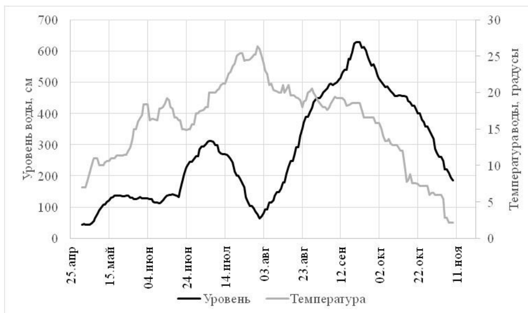
Рис. 2.13. Сезонная динамика уровня и температуры воды в бассейне Амура по створу г. Хабаровск в 2020 г.
