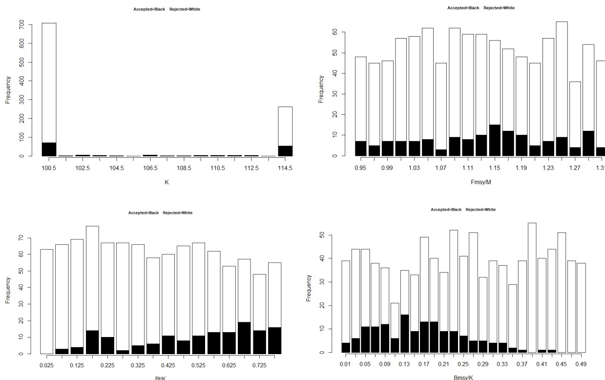
Рис. 3.25. Принятые и отвергнутые параметры для построения траекторий биомасс.
