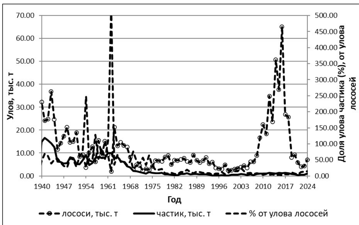
Рис. 2.5. Уловы пресноводных рыб и лососей в р. Амур за период с 1937 г. по 2024 г.
