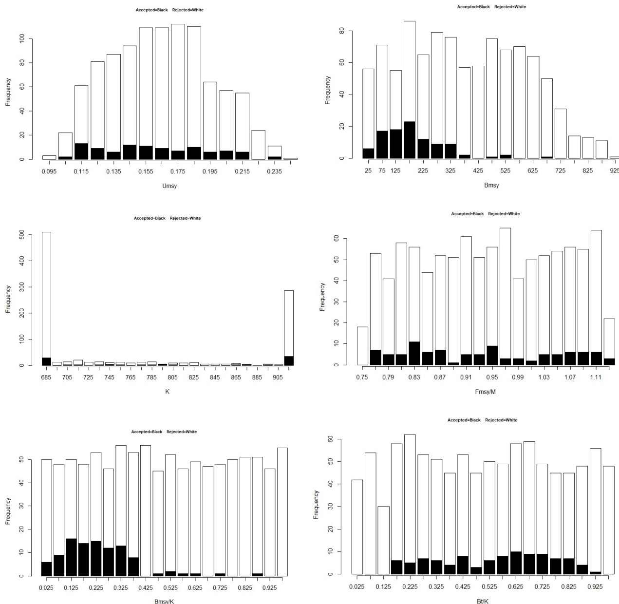
Рис. 3.16. Принятые и отвергнутые параметры для построения траекторий биомасс.
