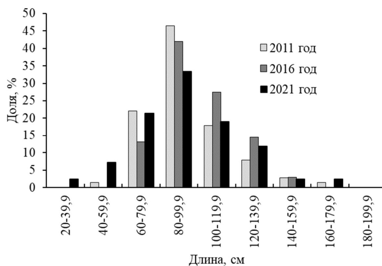
Рис. 6.4. Распределение амурского осетра по длине, лиман Амура
