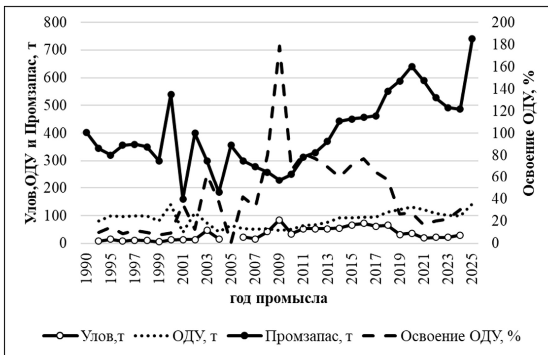
Рис. 3.9. Динамика промысла, ОДУ, уловов (т) и освоения ОДУ (%) сазана в пределах Хабаровского края и ЕАО
